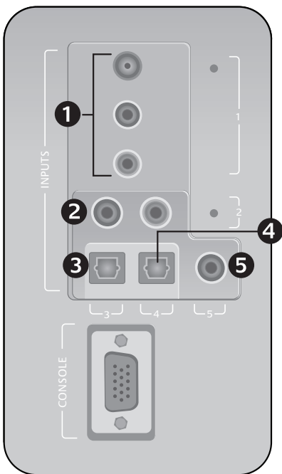
Painel posterior do subwoofer
